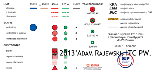
Plan sieci elektroenergetycznej najwyższych napięć
